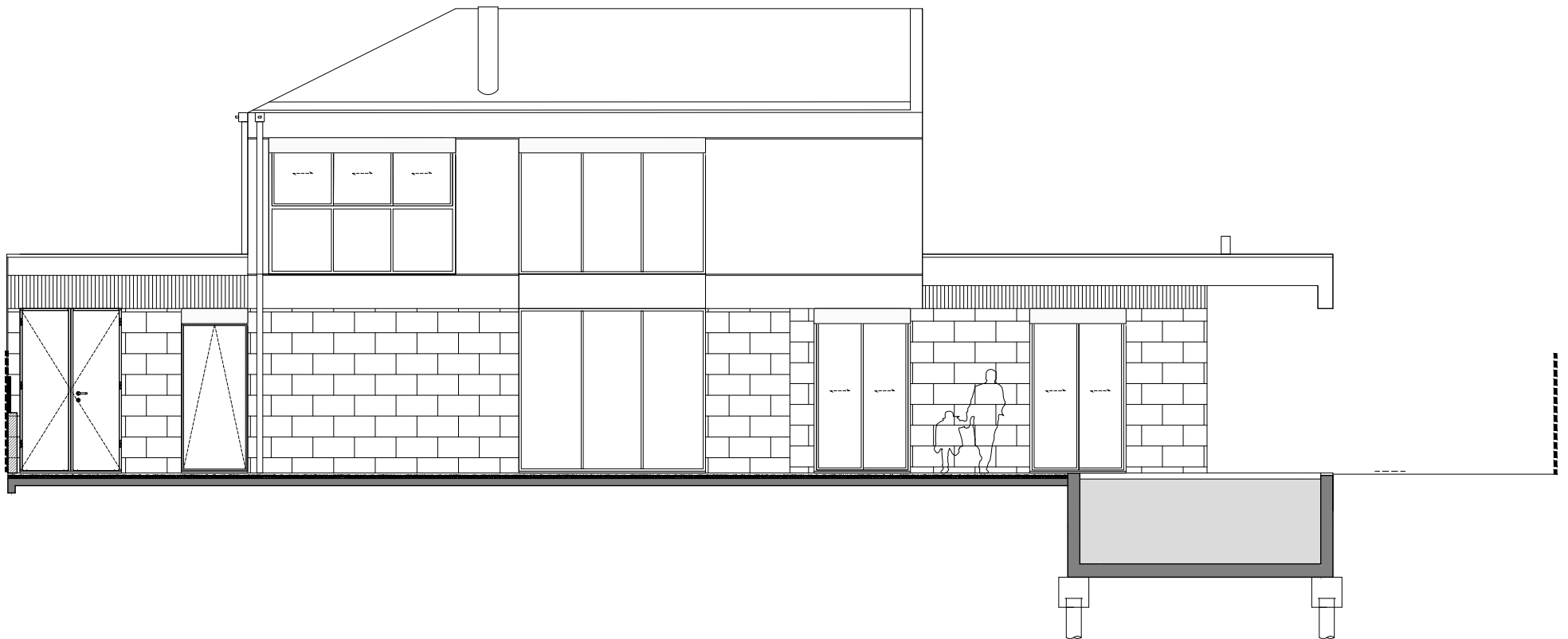
façade Ouest / échelle : 1/100
