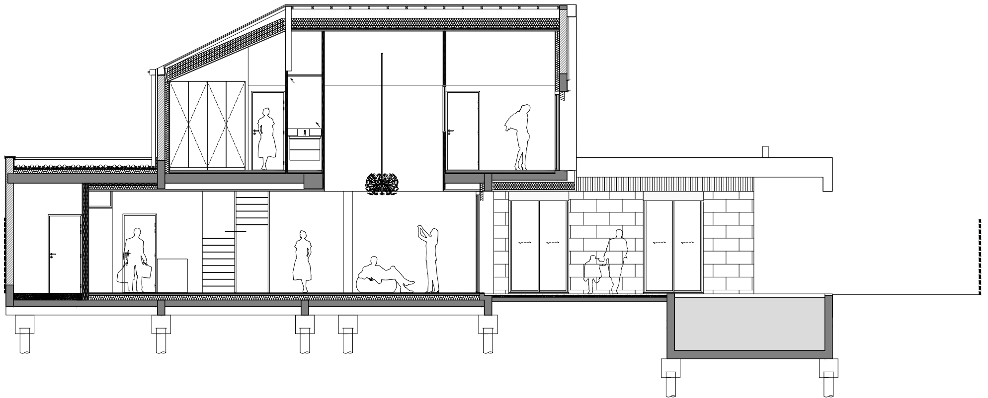
coupe longitudinale / échelle : 1/100
