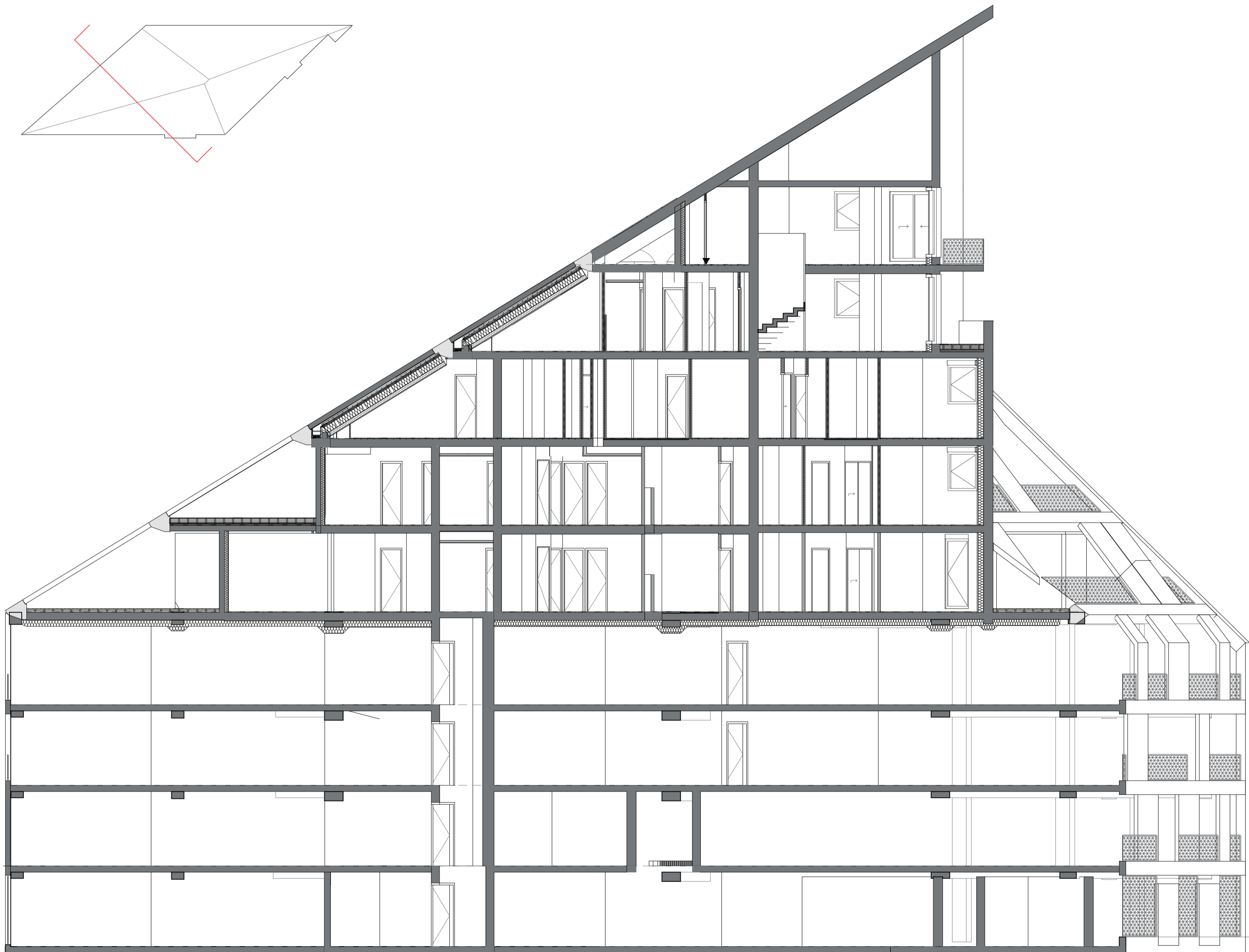
COUPE DE PRINCIPE // PENTE A 31.5°
