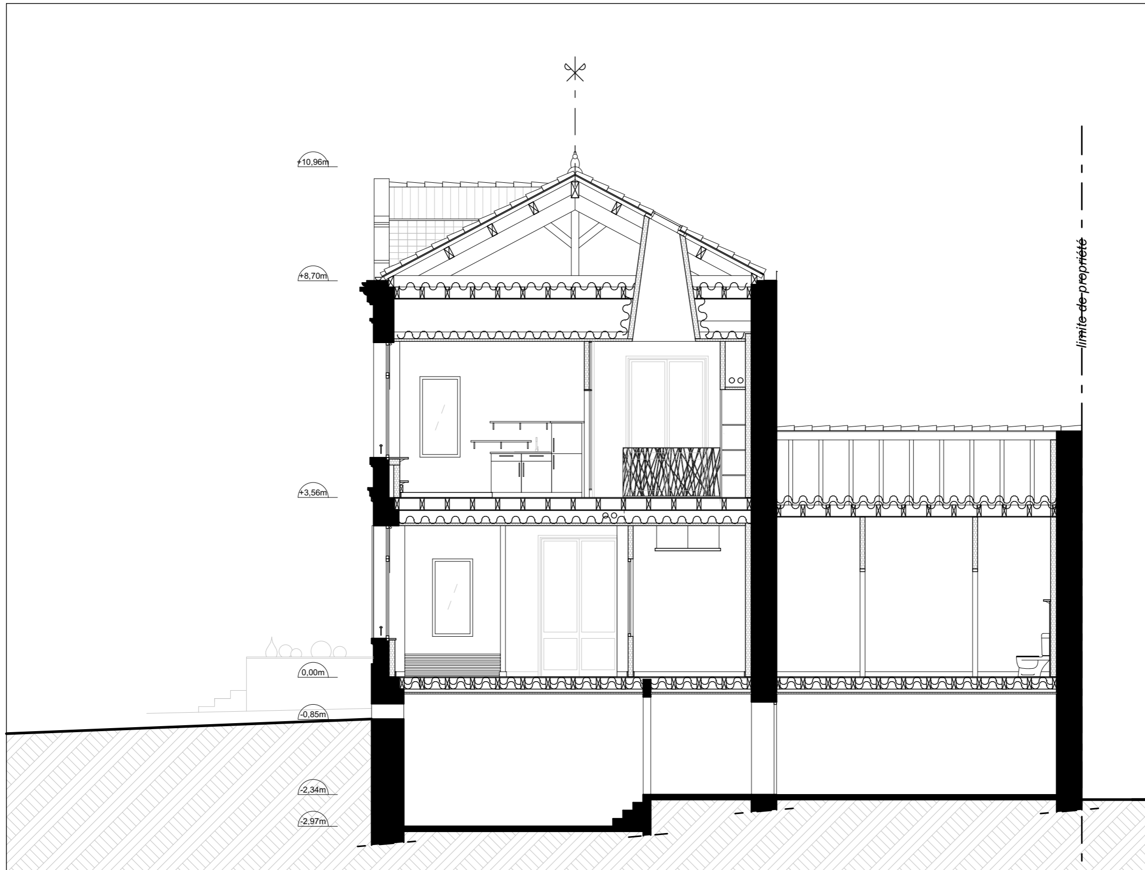
PROJET - COUPE AA - éch : 1/75
