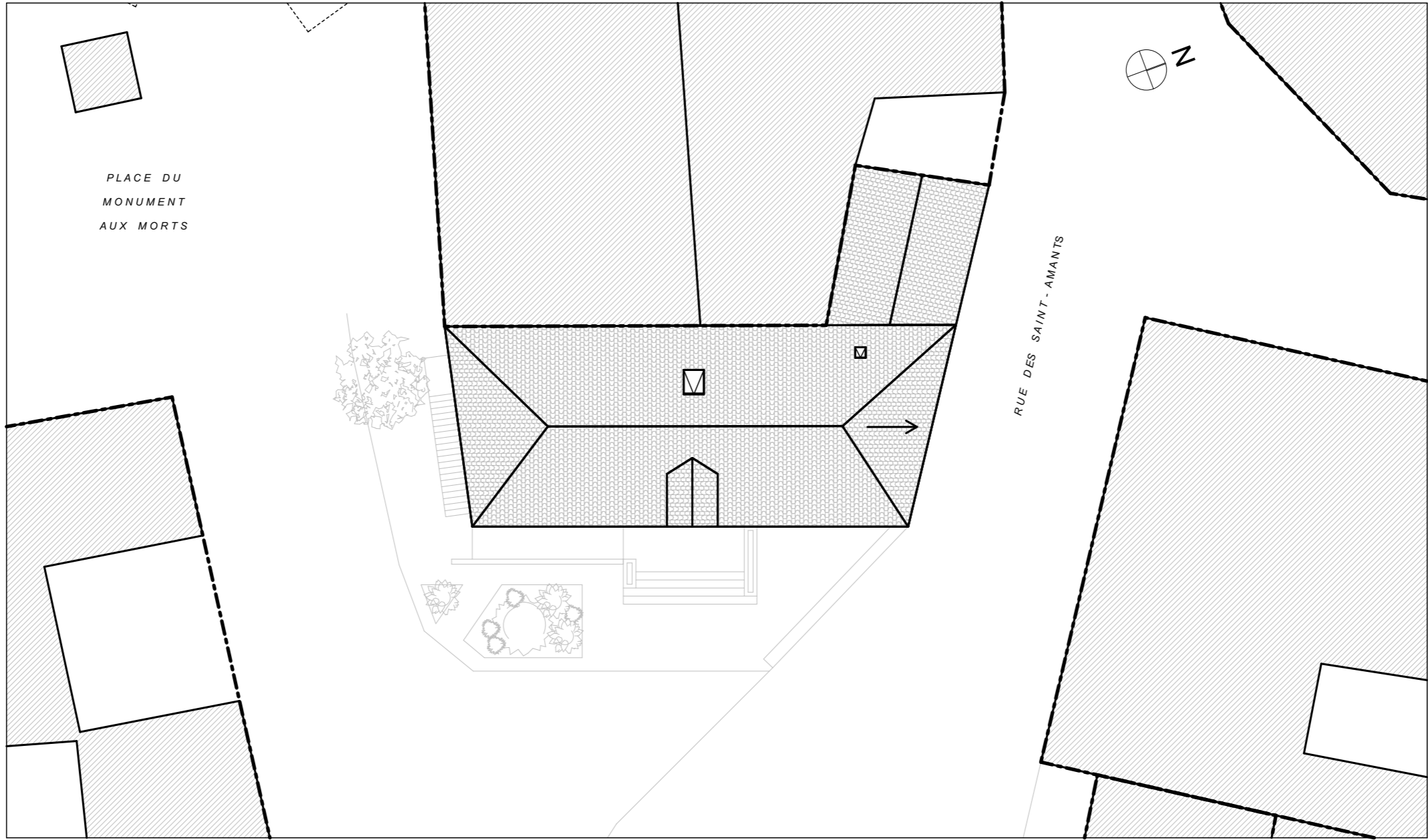
ETAT DES LIEUX - PLAN MASSE - éch : 1/200
