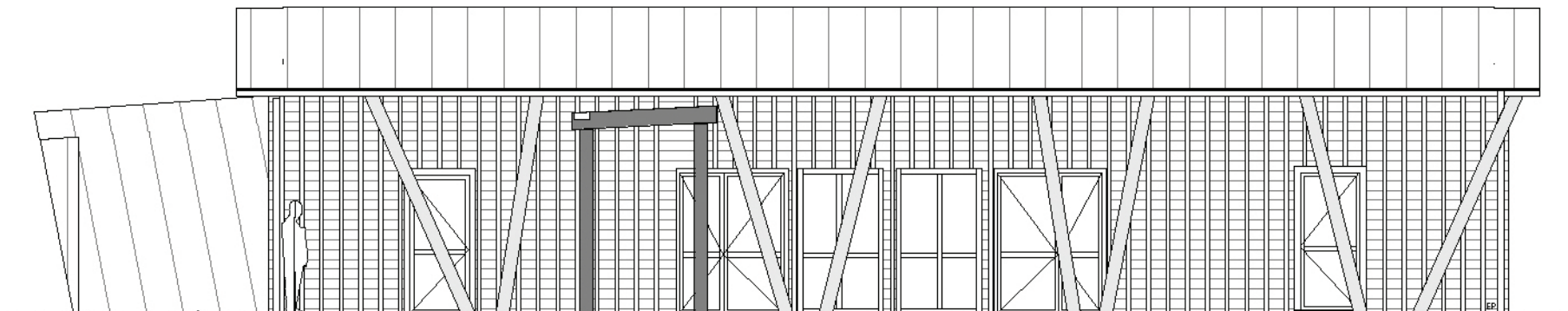
ALLIANCE FORÊT BOIS : FACADE NORD-OUEST - 1 : 100
