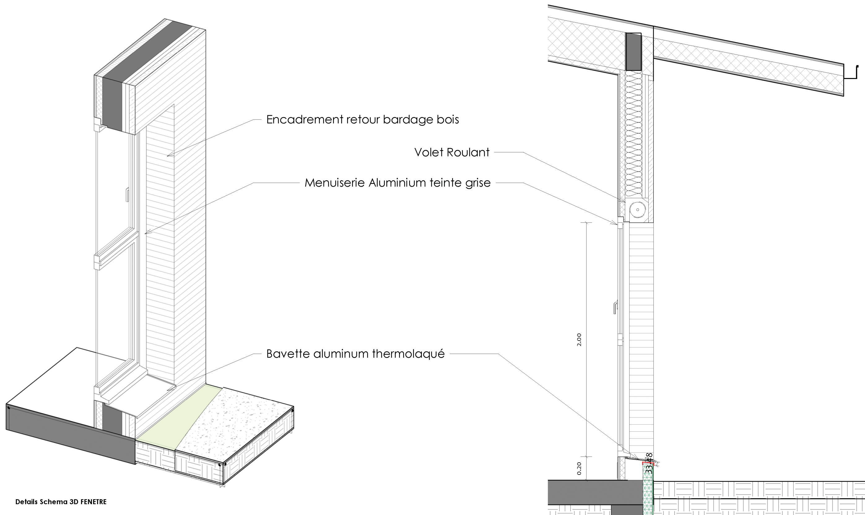
Coupe Fenêtre
