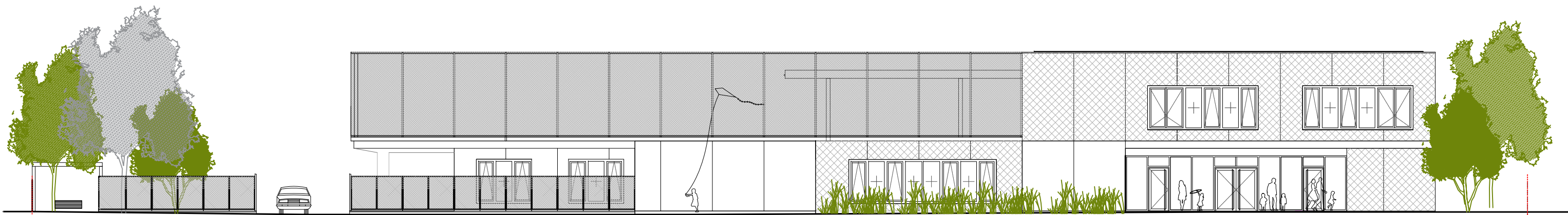
ELEVATION EST - FACADE PRINCIPALE SUR RUE FRANCOISE DOLTO - ECH: 1/200
