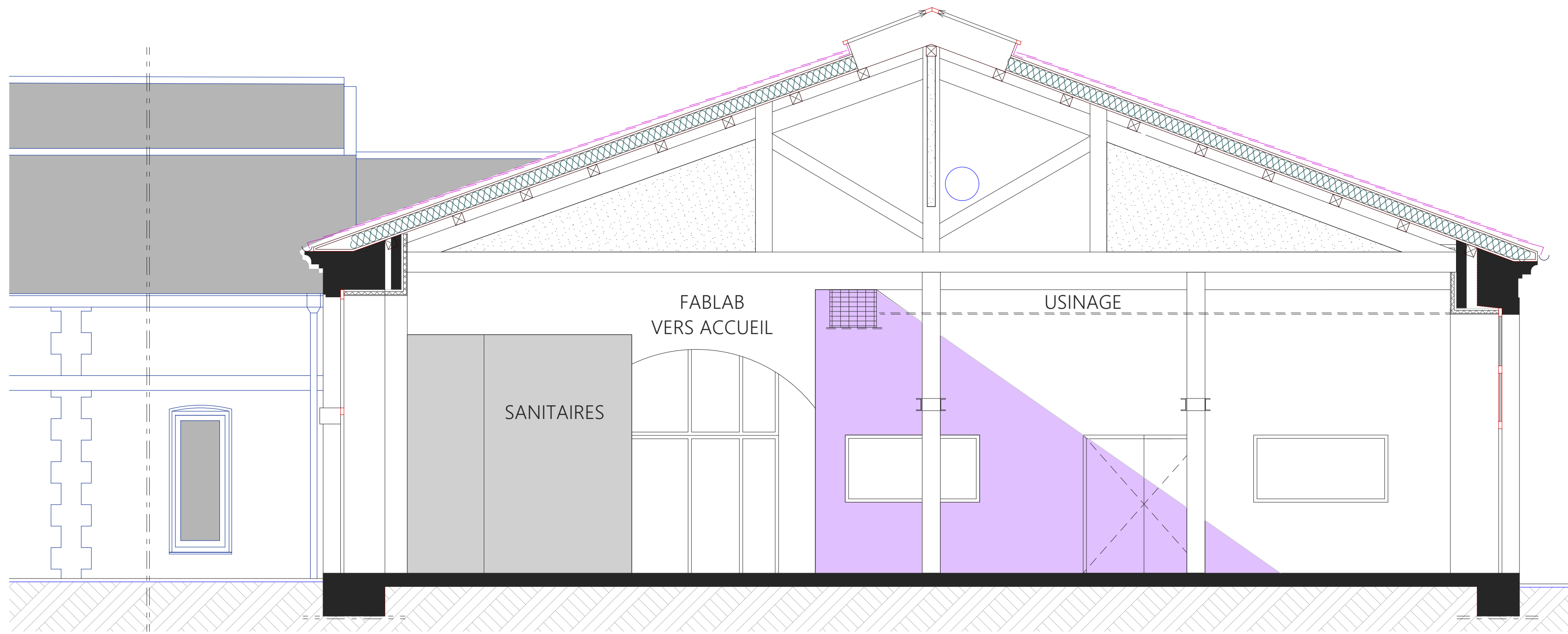
COUPE SUR ATELIER DU TECHNOPOLE
