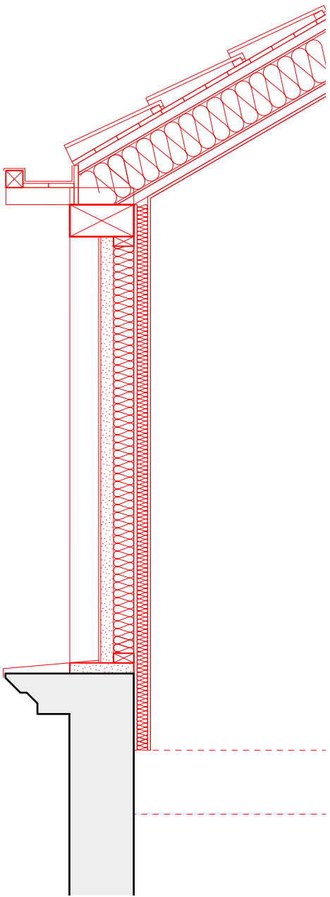
Coupe sur mur plein
