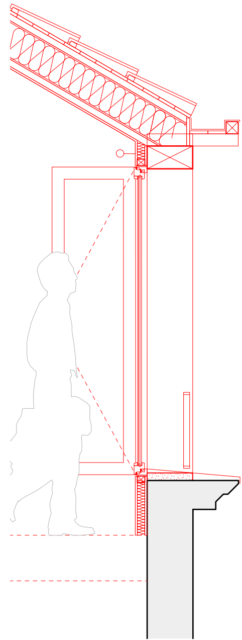
Coupe sur ouverture
