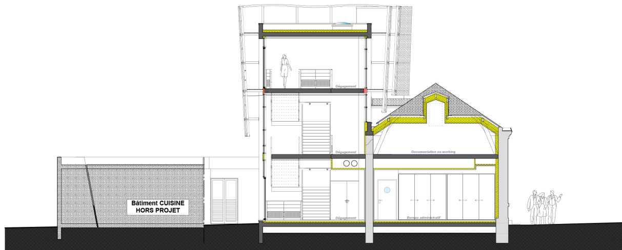
COUPE BB ECH: 1/100
