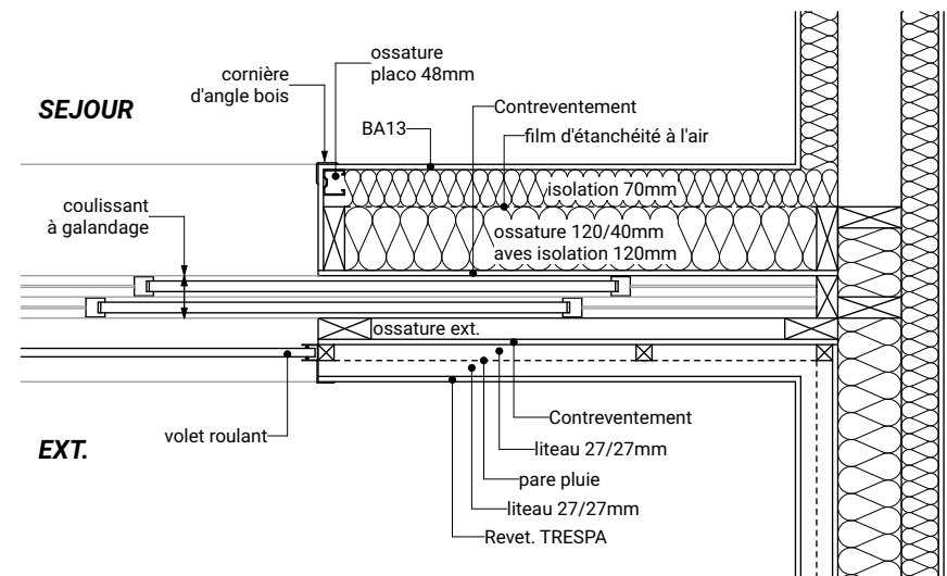
COUPE DE DETAIL SUR MUR DU SEJOUR
