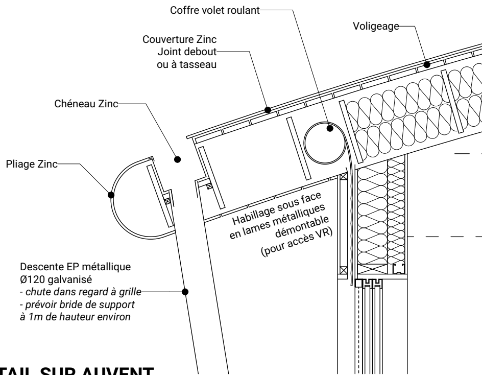
DETAIL SUR AUVENT
