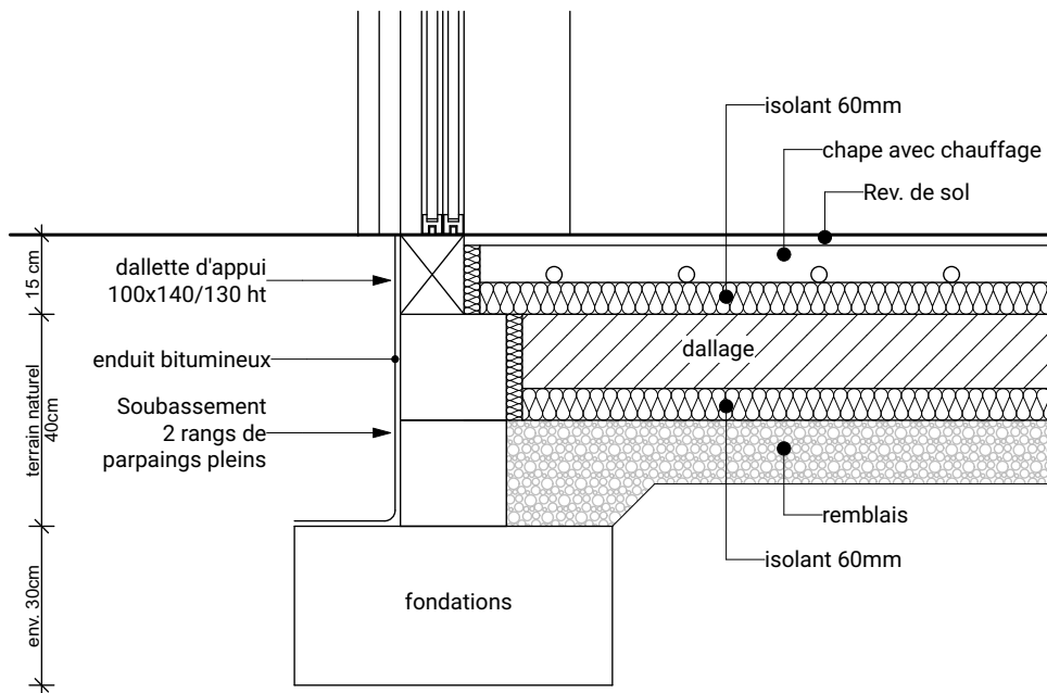
DETAIL SUR DALLAGE
