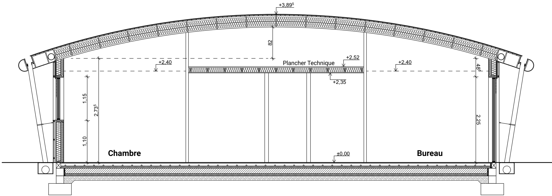
PRINCIPE DE COUPE SUR COIN NUIT
