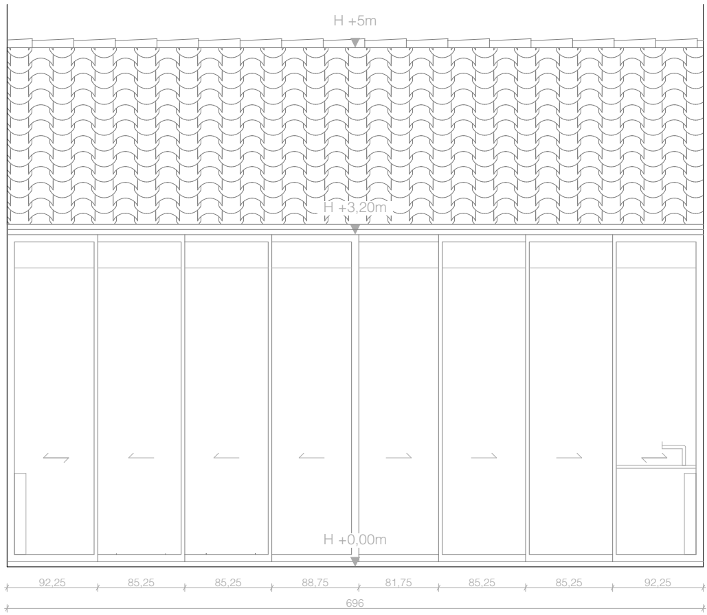
FAÇADE_PROJET_1/50
