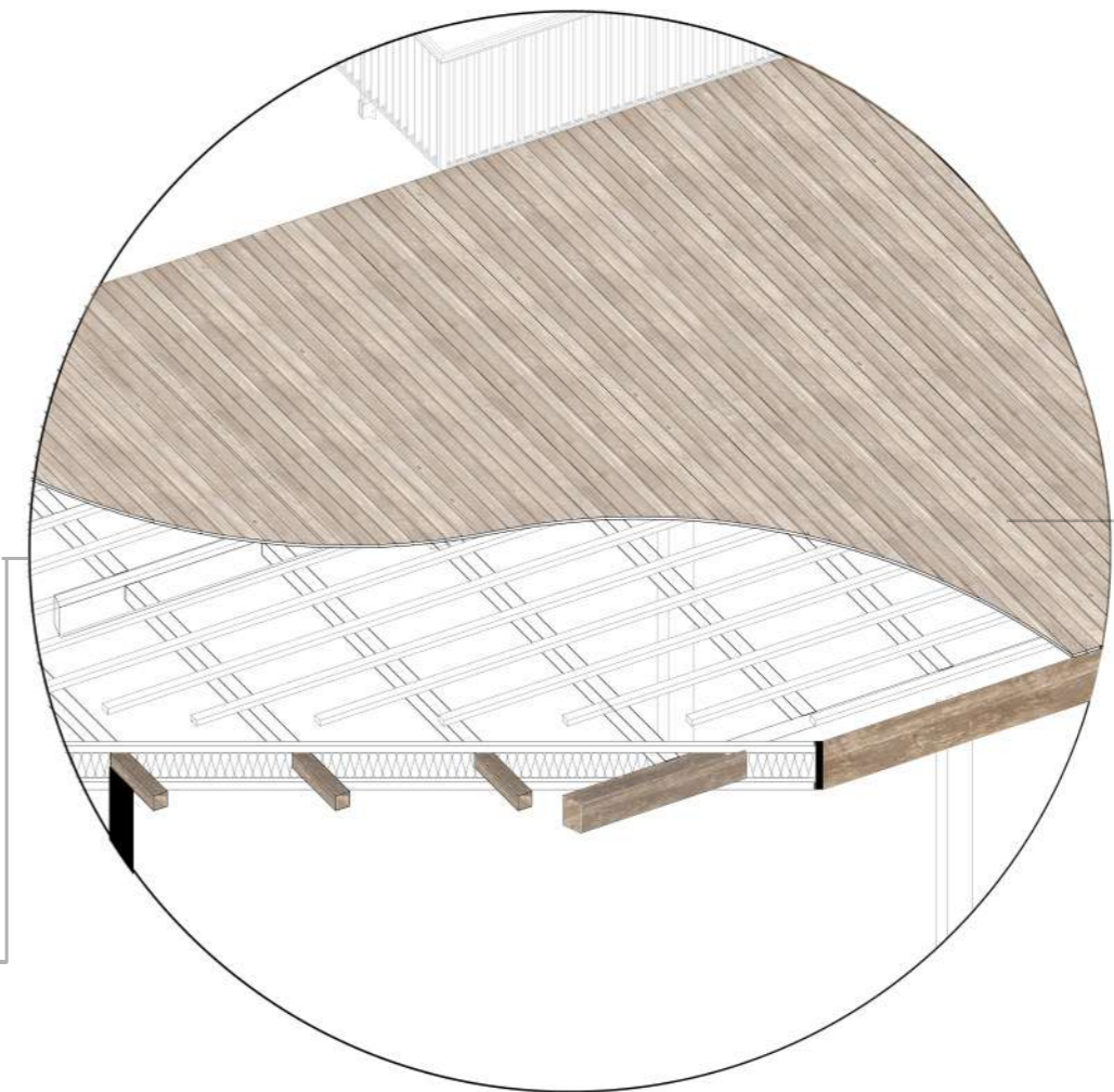
DETAILS CONSTRUCTIFS
