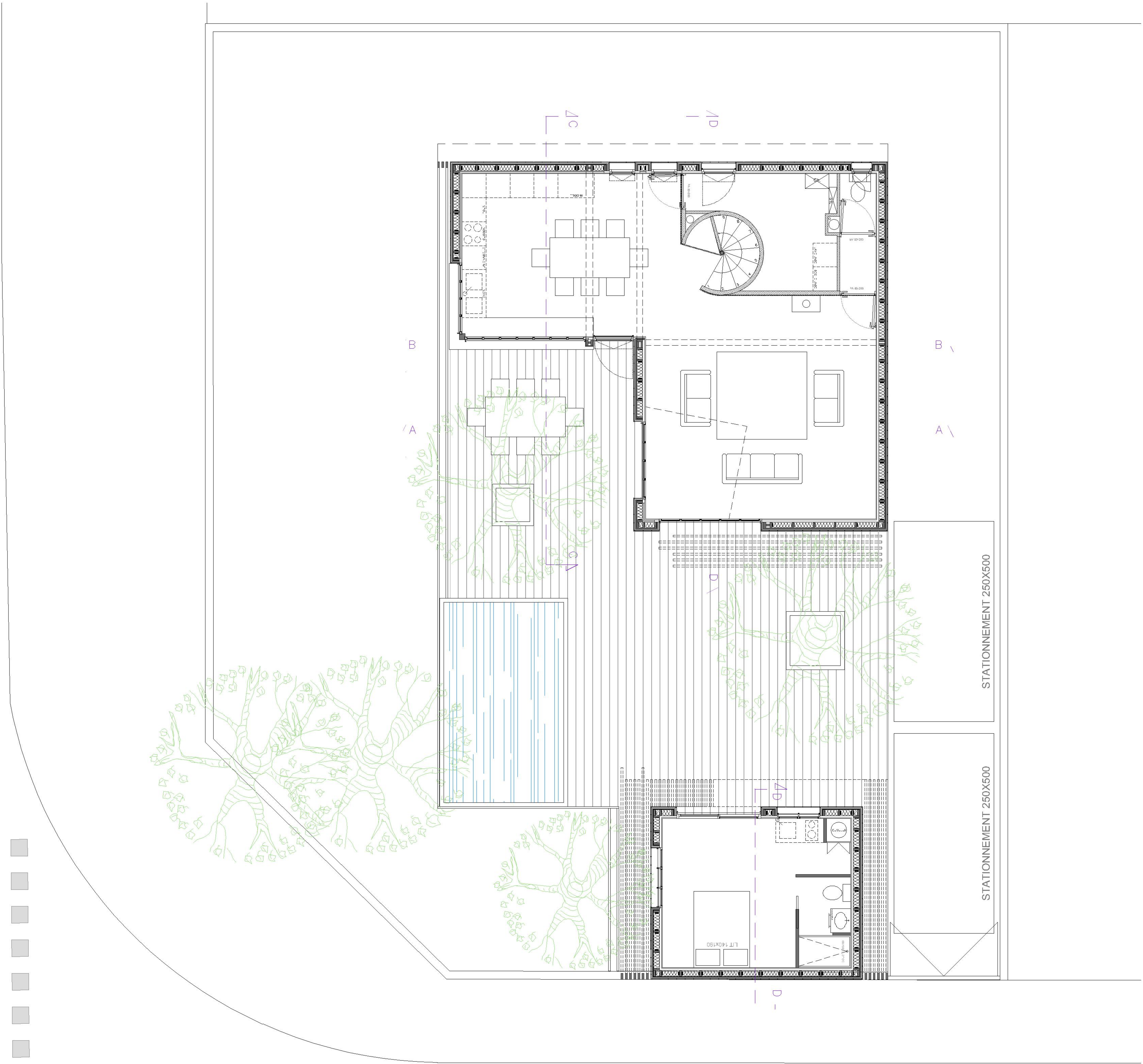
PLAN RDC
