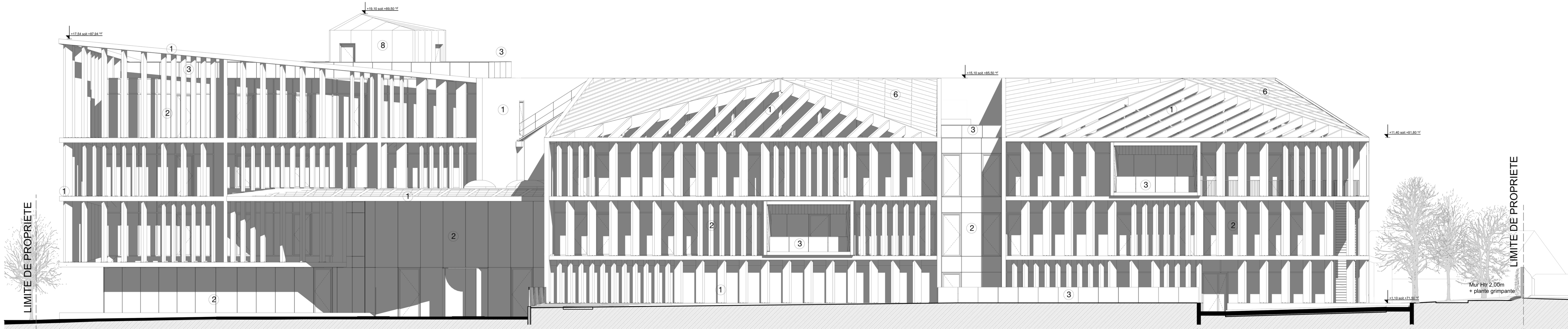
Façade Ouest
