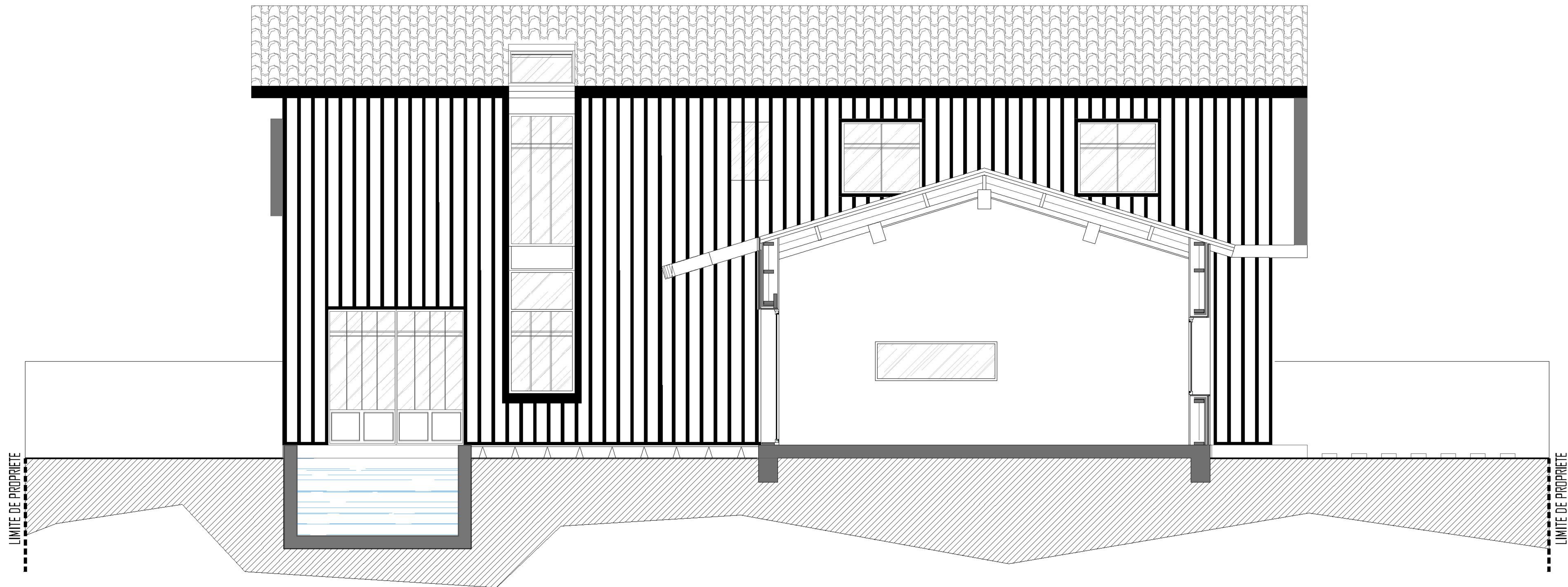
COUPE B-B
