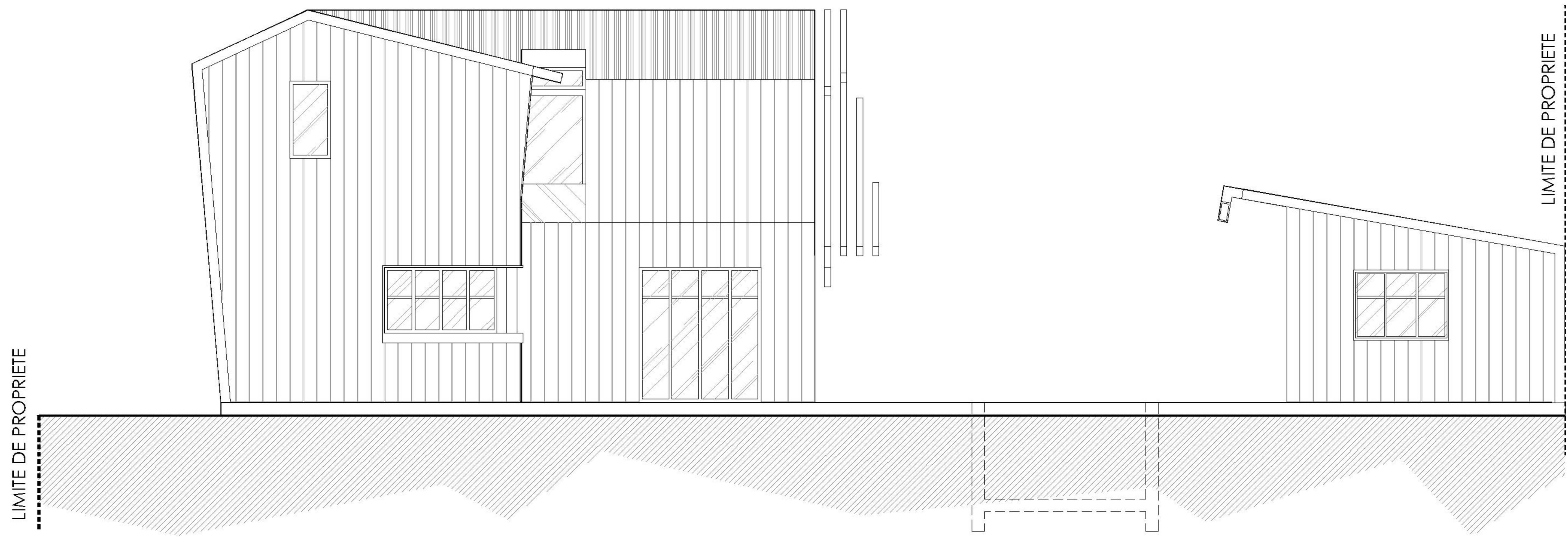
FAÇADE SUD-OUEST
