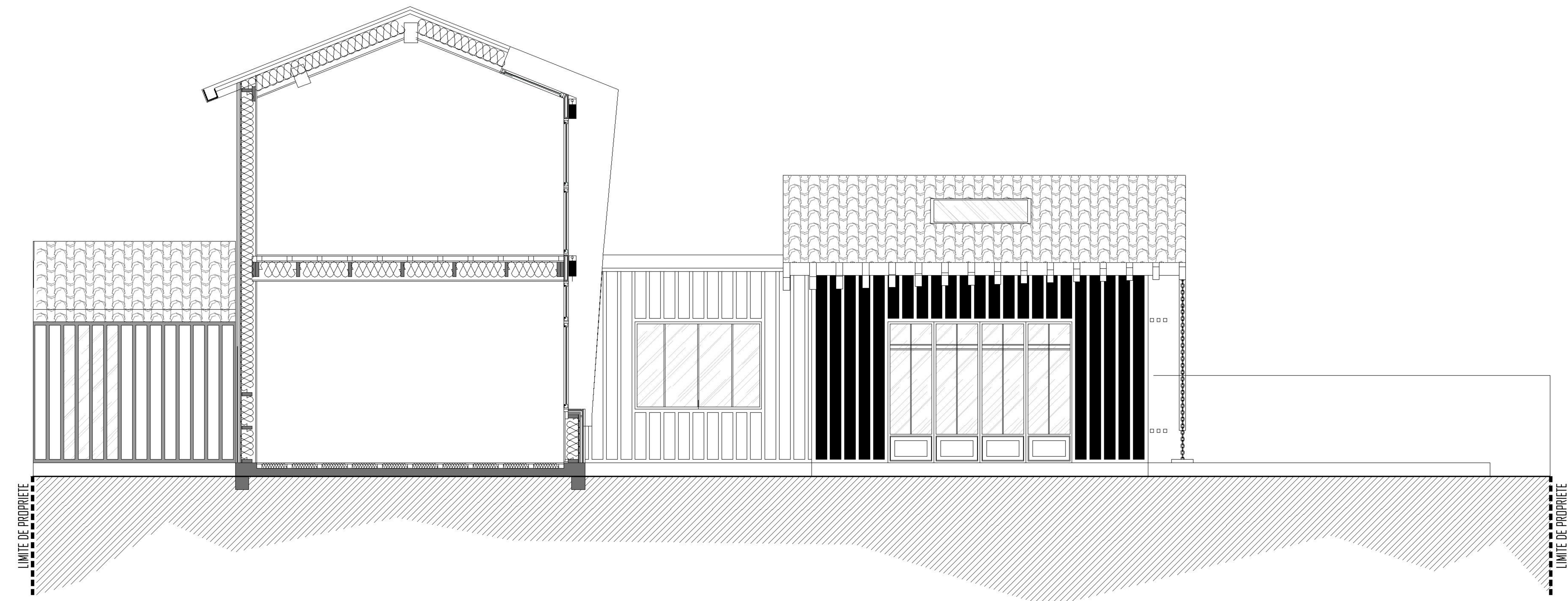
COUPE A-A
