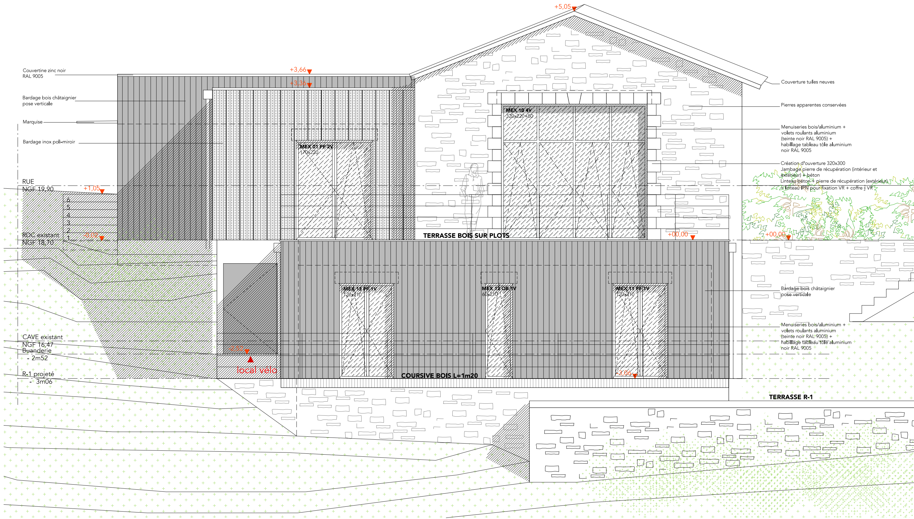
Façade Nord ouest
