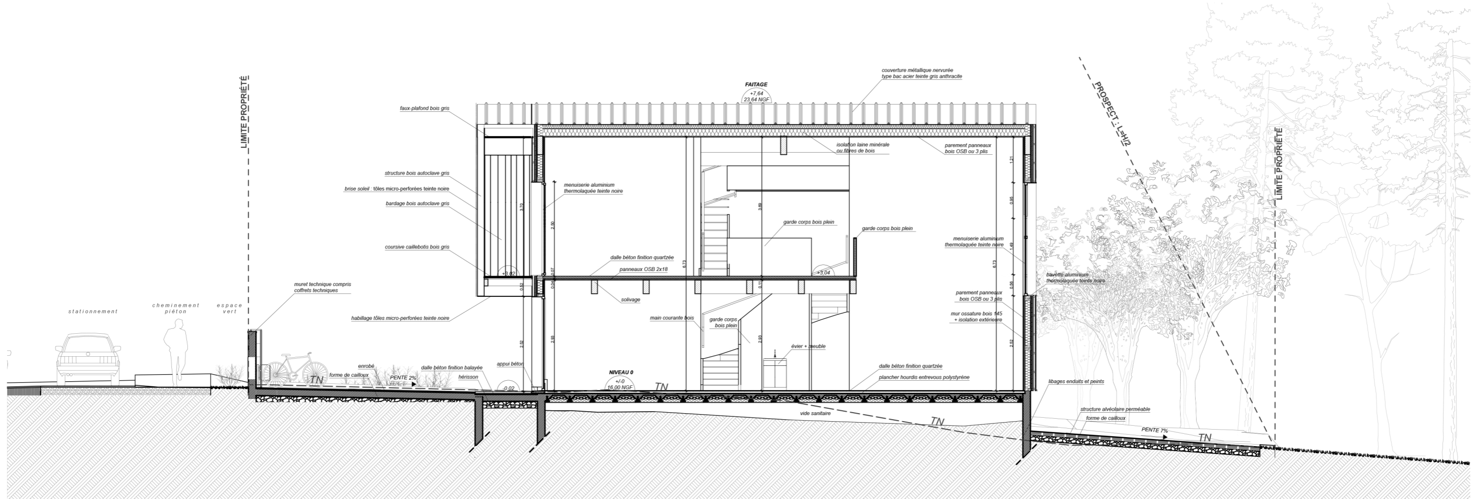
COUPE A
