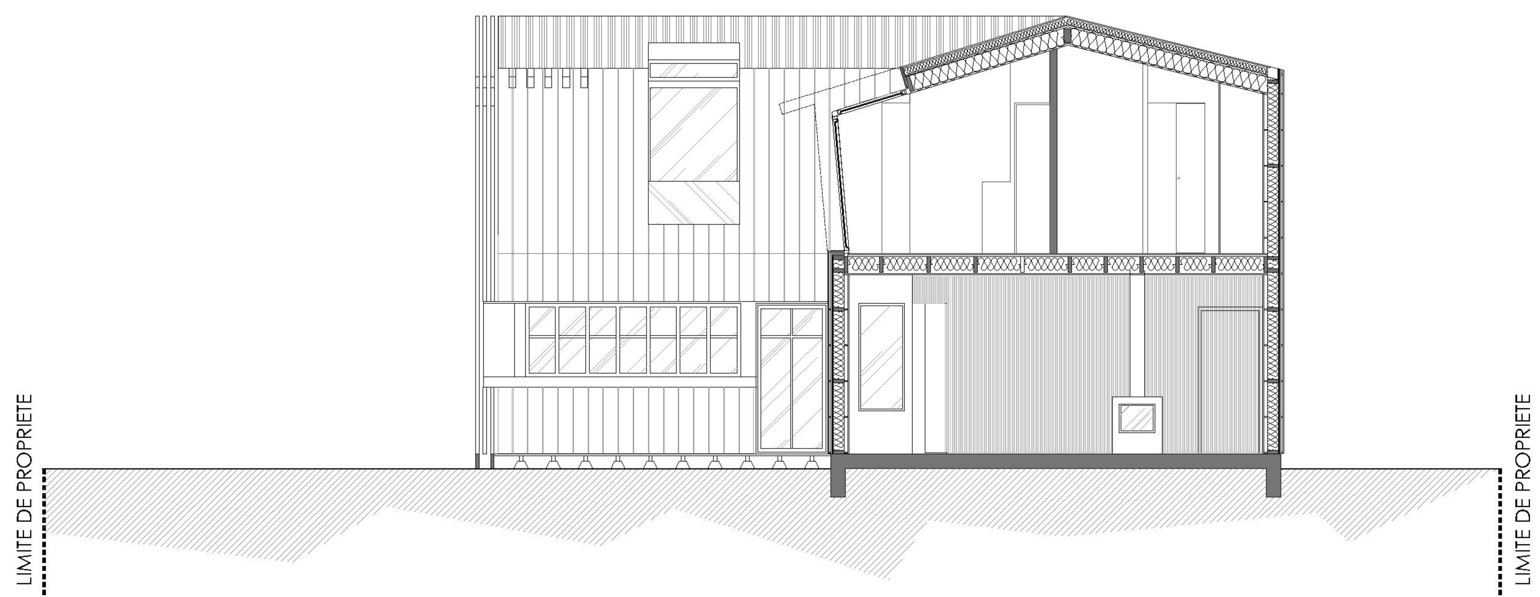
COUPE B-B
