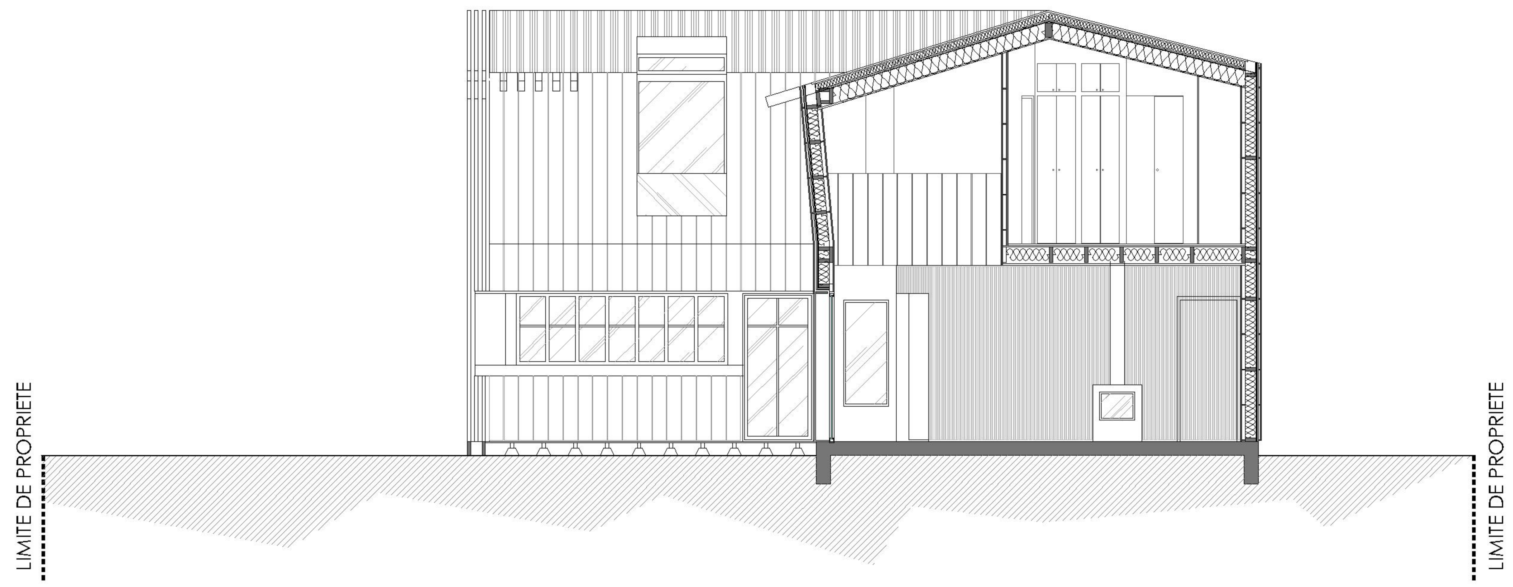
COUPE A-A
