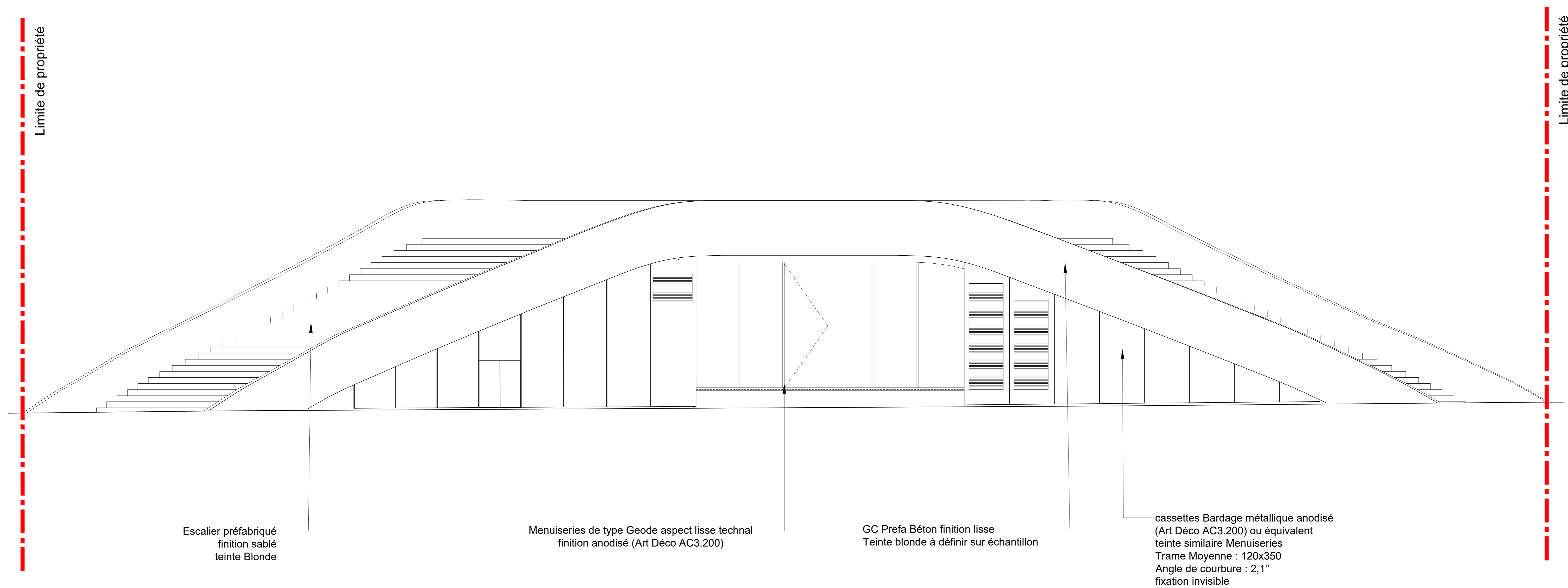
ELEVATIONS OUEST
