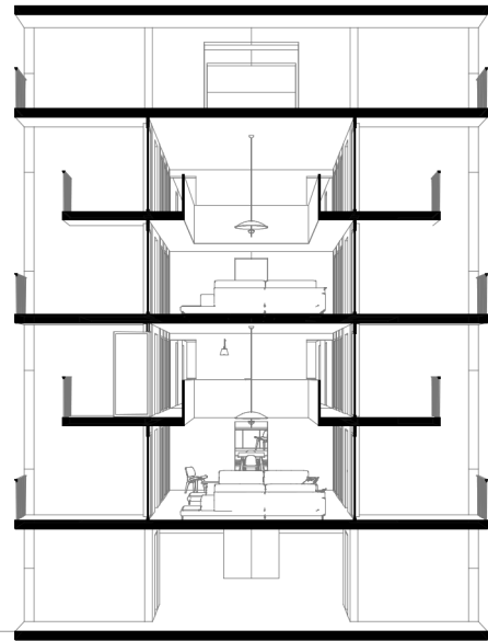
Coupe transversale sur les espaces partagés à 16 habitants [échelle 1/200]
