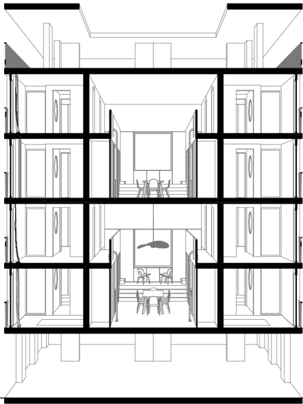
Coupe transversale sur les chambres privées et sur les espaces partagés à 8 habitants [échelle 1/200]
