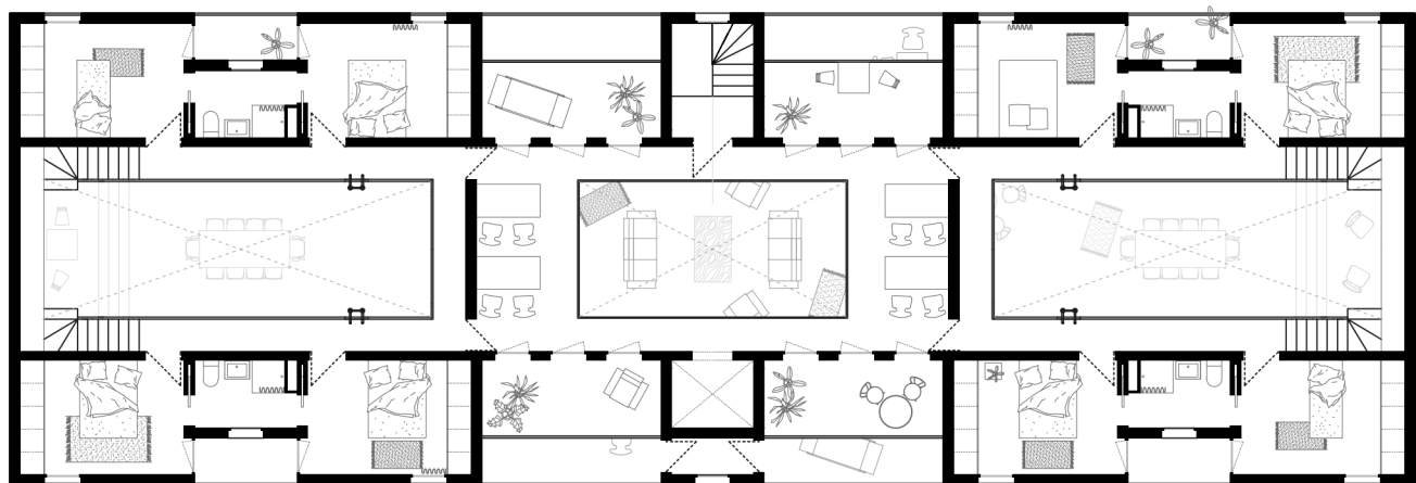
Plan étage courant, niveau haut d'habitat partagé [échelle 1/200]
