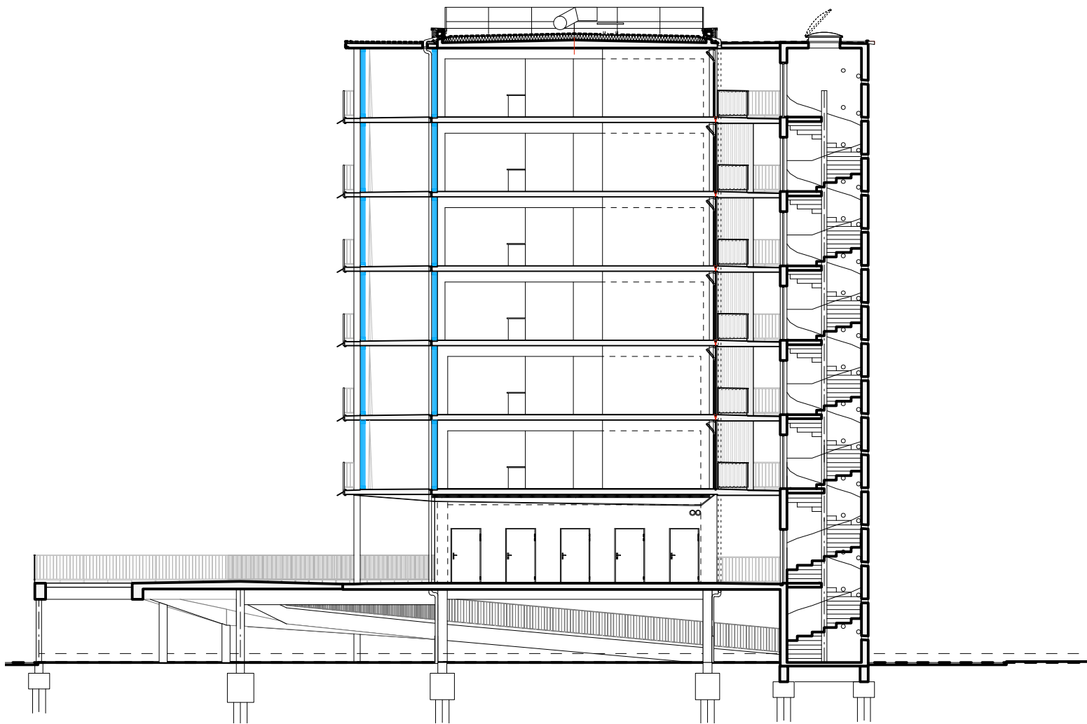
coupe transversale ech. 1/200°
