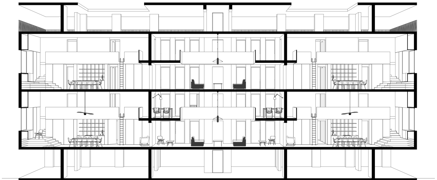
Coupe longitudinale [échelle 1/200]
