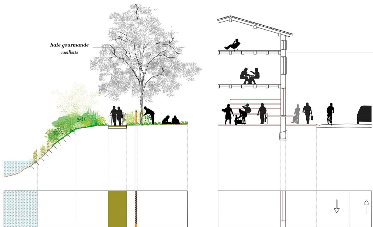
Berge clayonnages saules et graviers Ripisylve héliophytes vivaces de mi-ombre Chemin de halage reconstitution Vergers traversées publiques rétrogradées à la ville et parcelles privées avec clôtures basses
