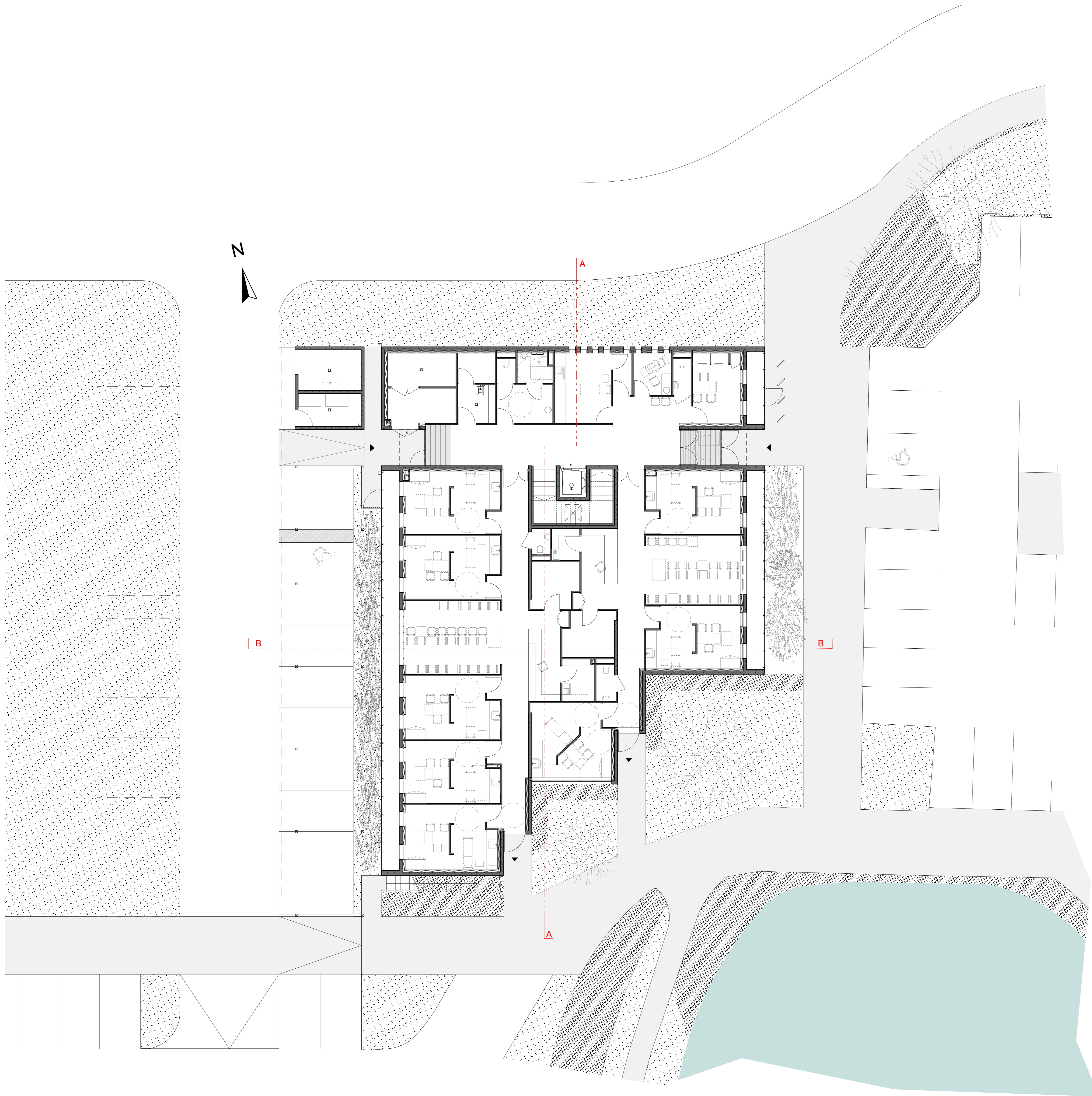
plan rez-de-chaussée
