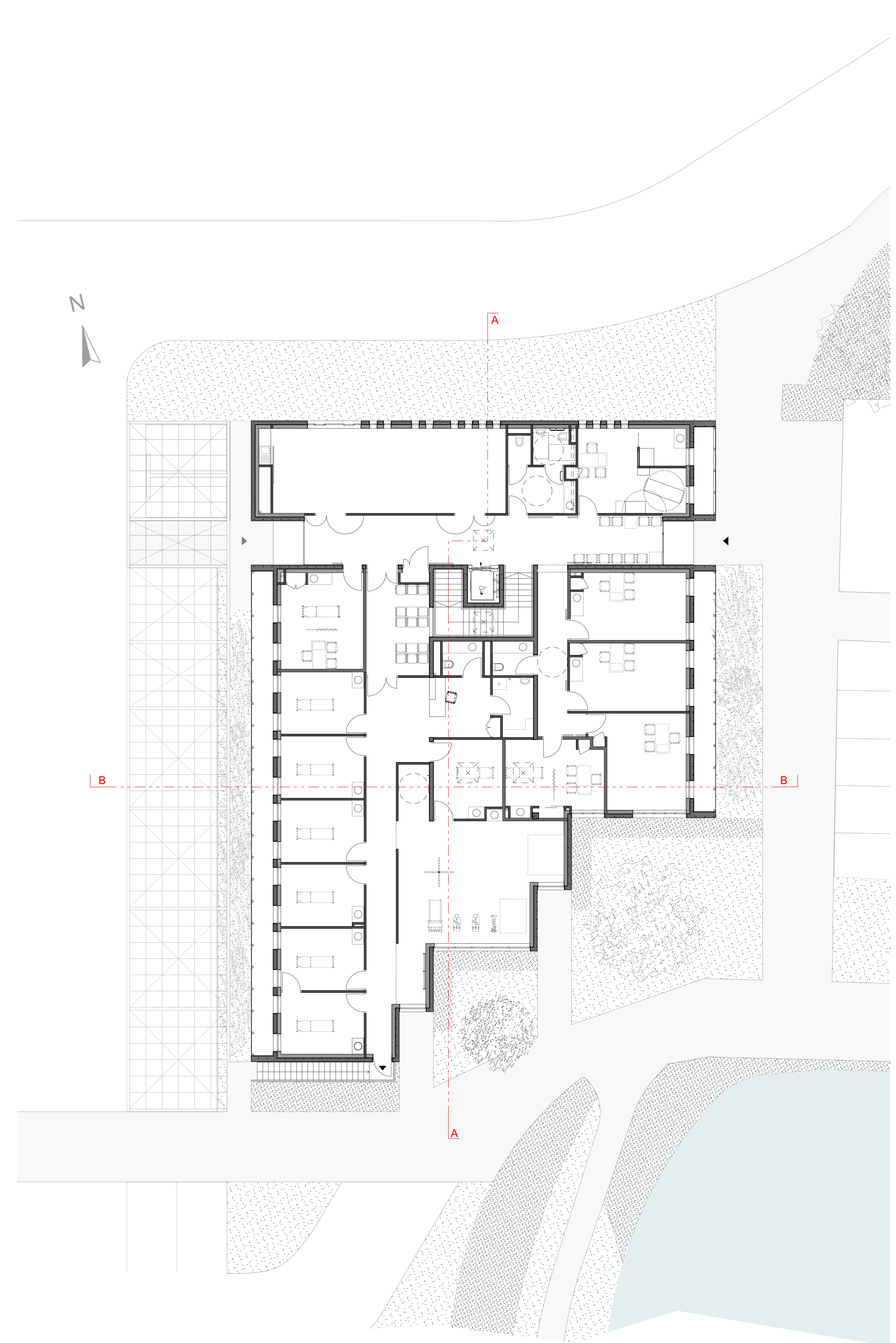
plan premier étage
