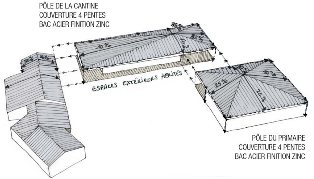
PÔLE DE LA MATERNELLE PROLONGEMENT TOITURE EXISTANTE COUVERTURE DEUX PENTES MÊME TUILE QUE L'EXISTANT
