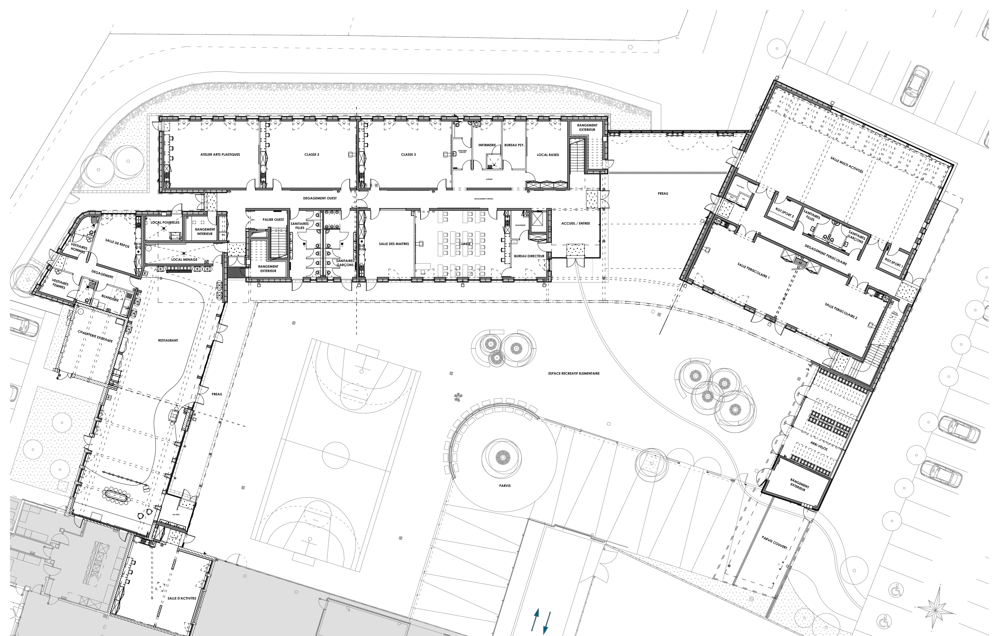
PLAN REZ DE CHAUSSEE
