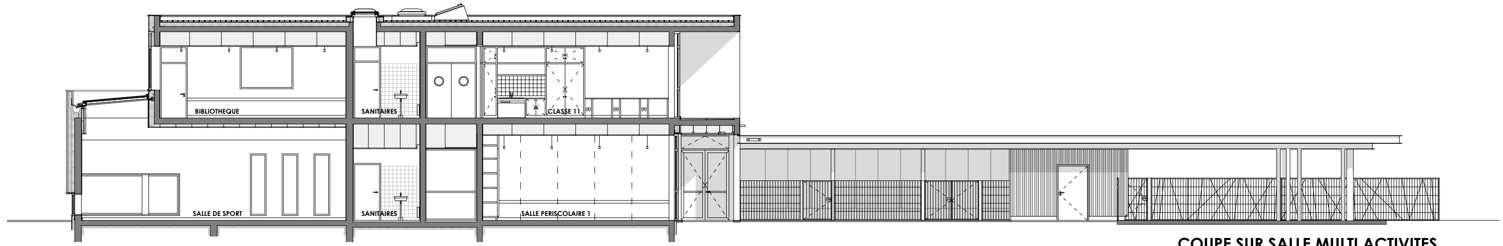
COUPE SUR SALLE MULTI ACTIVITES
