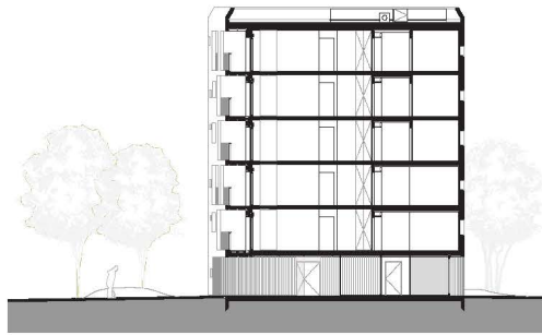
Coupe BB' 0 5 10 20 m.
