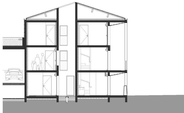
COUPE TRANSVERSALE MAISON INDIVIDUELLES 0 2 4
