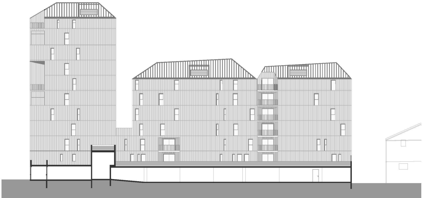
ELEVATION NORD OUEST
