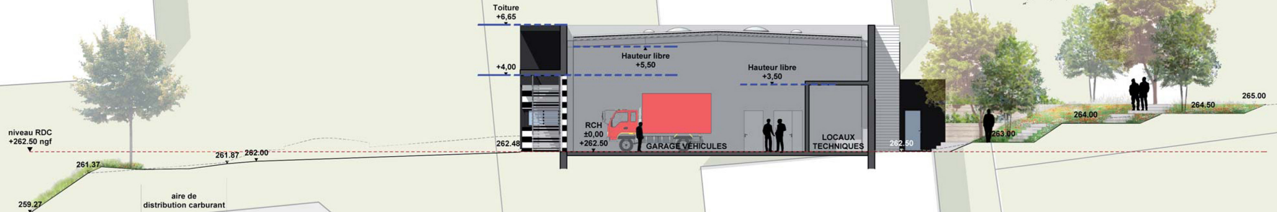
COUPE TRANSVERSALE BB' SUR GARAGE VEHICULES échelle : 1/200°
