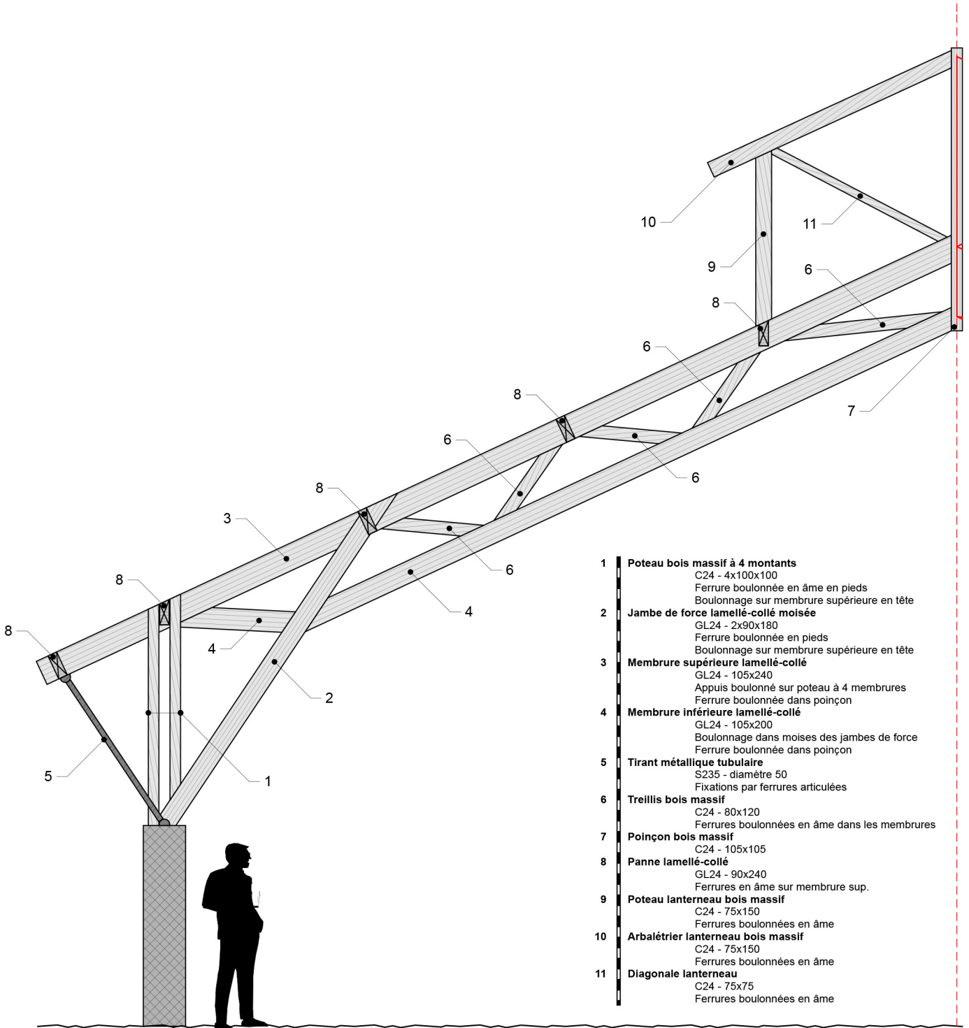
COUPE SUR PORTIQUE PRINCIPAL - 1:50 e
