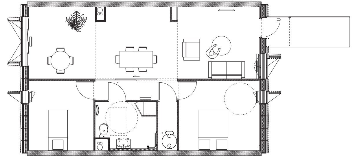
plan type [échelle 1:100]
