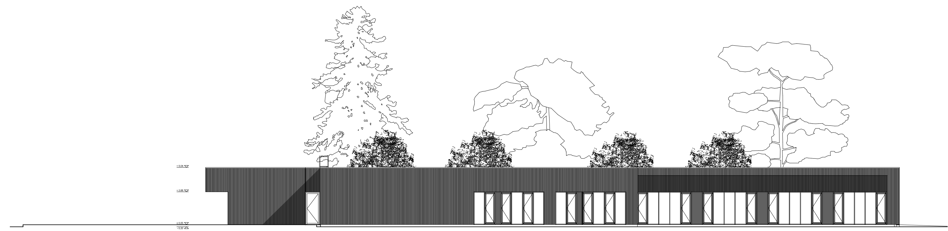
élévation sud
