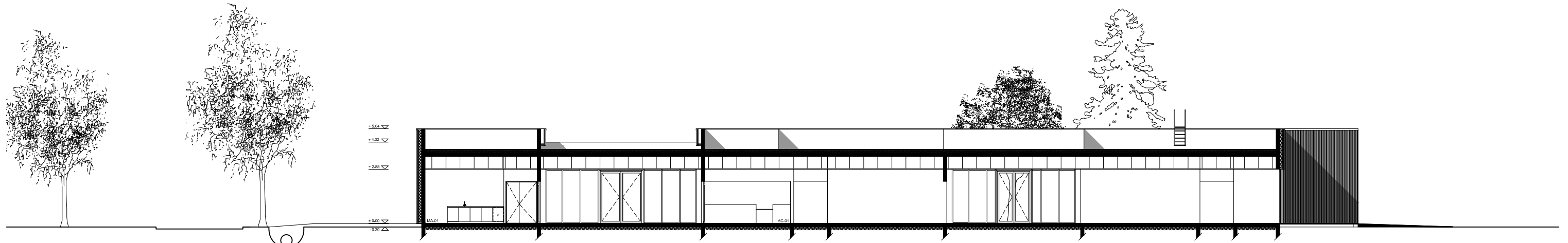
coupe CC
