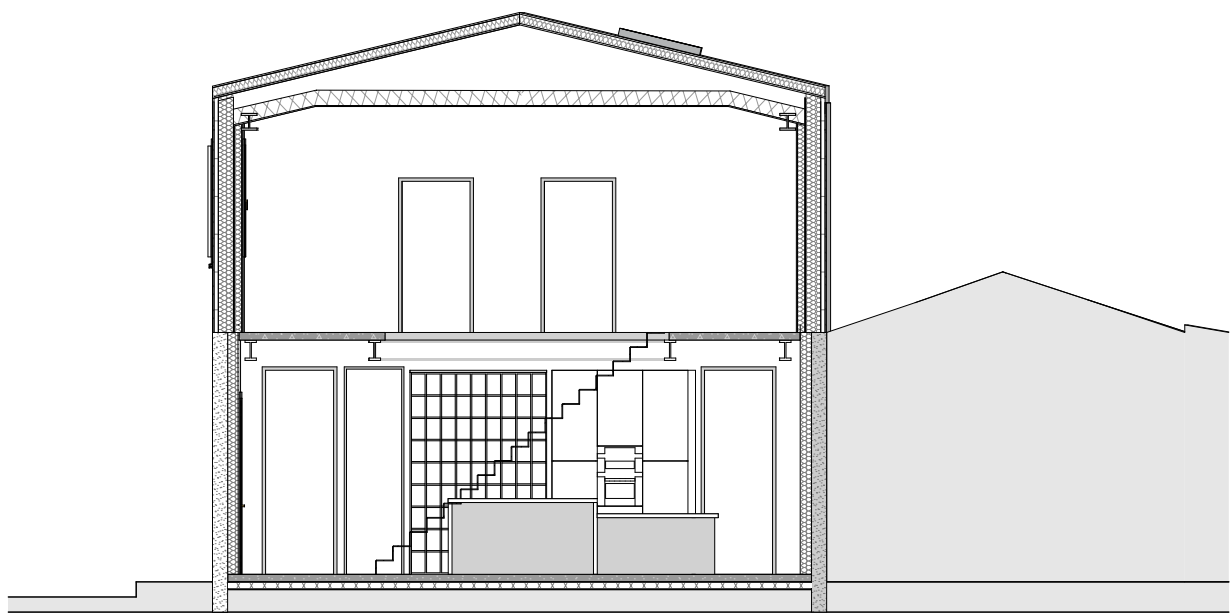
Coupe transversale
