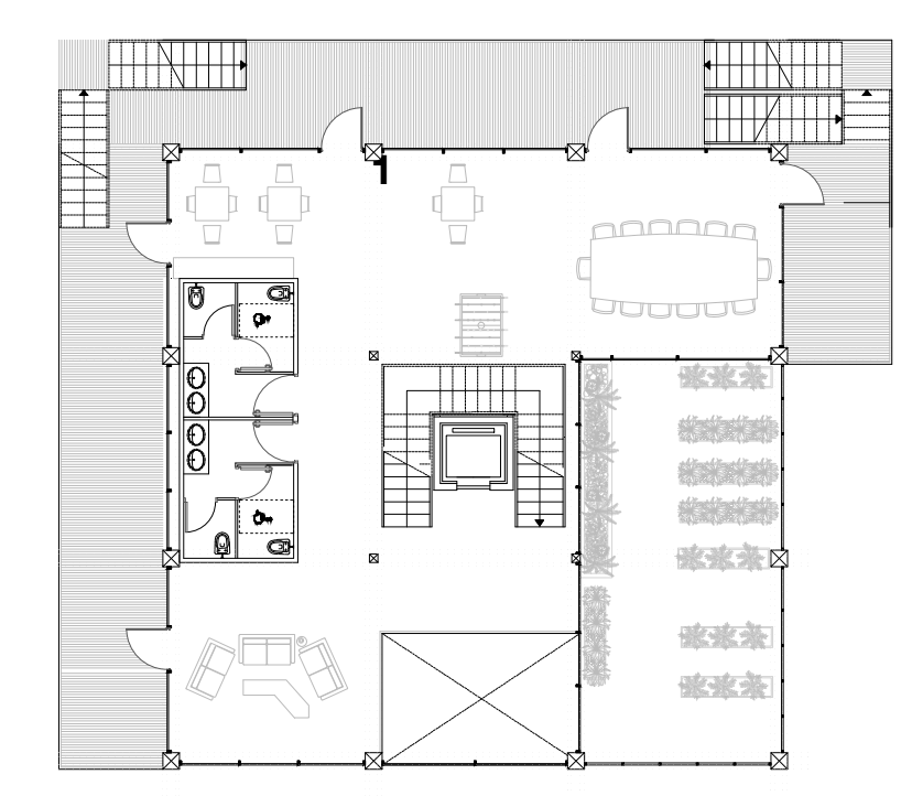
Plan R+1 1:200 1. Espace associatif
