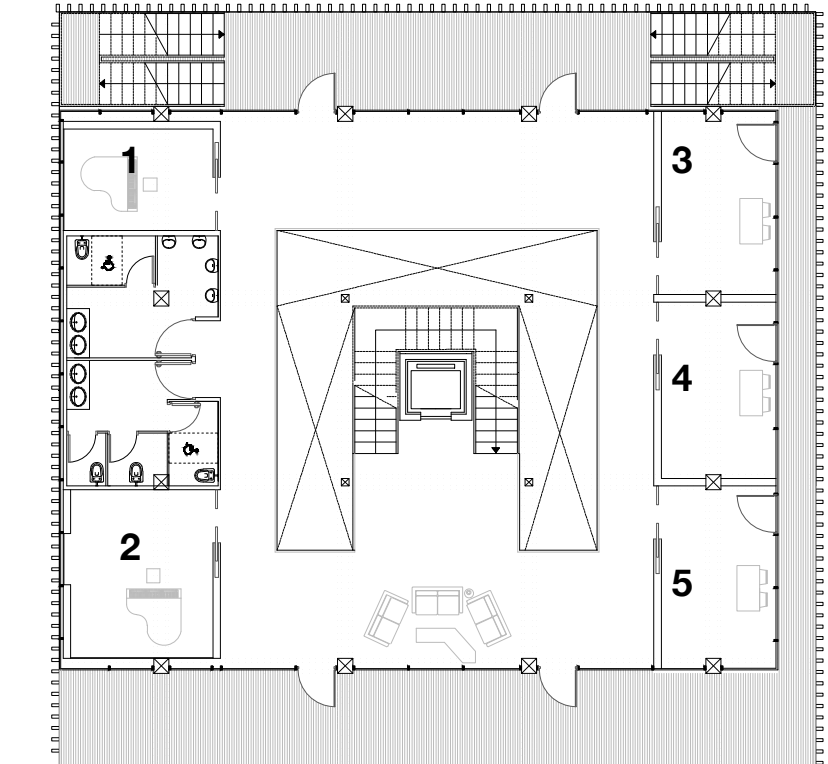
Plan R+5 1:200 1. Studio de musique 2. Studio de musique 3. Salle de cours 4. Salle de cours 5. Salle de cours
