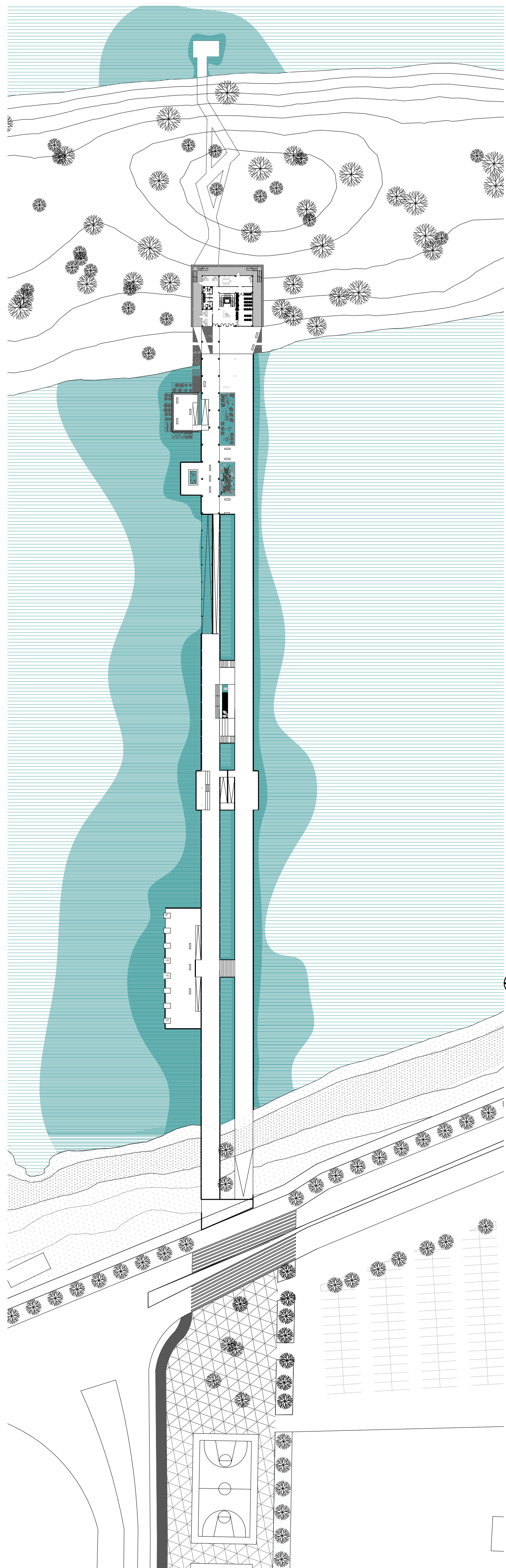
Plan masse du projet 1:1000
