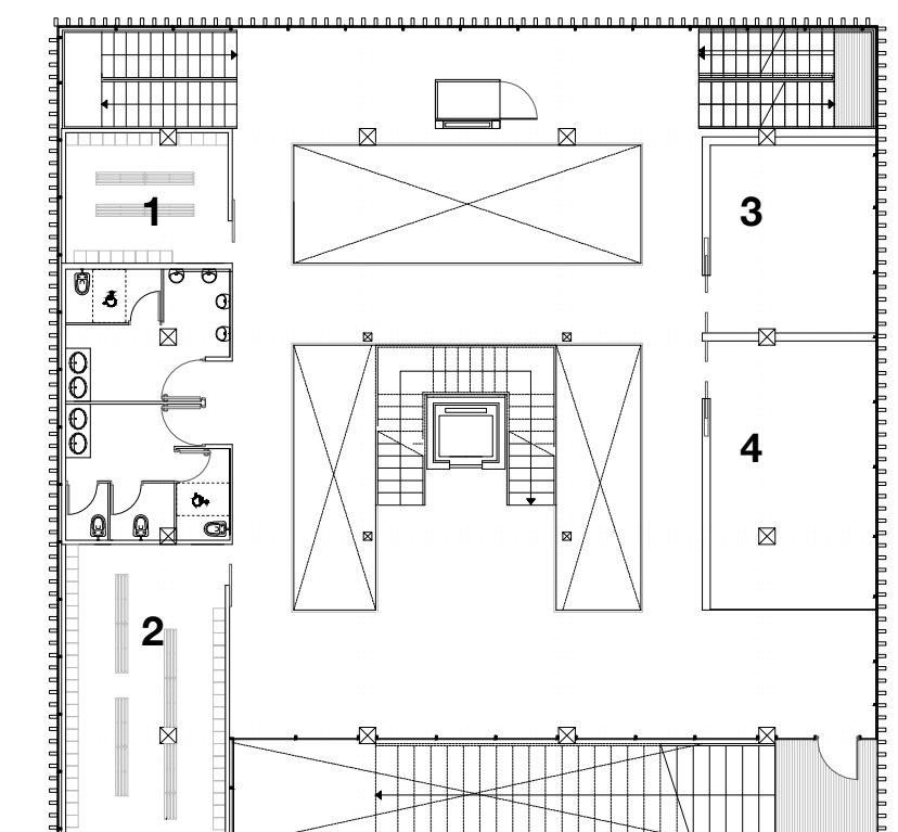
Plan R+6 1:200 1. Vestiaires H 2. Vestiaires F 3. Salle de cours 4. Salle de cours
