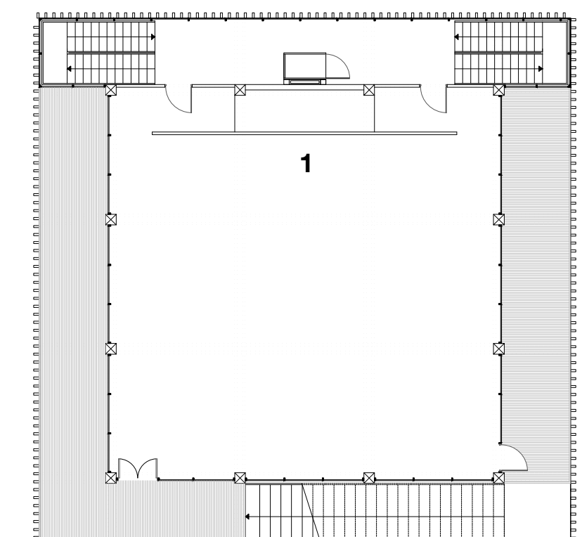
Plan R+7 1:200 1. Salle de danse / Yoga
